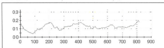
円周断面 (PV=0.152 \mu m RMS=0.031 \mu m)
