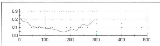
Y断面 (PV=0.174 \mu m RMS=0.042 \mu m)
